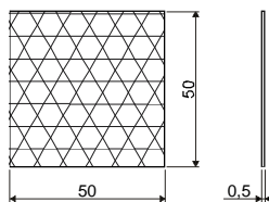
ODR50x50 F (samolepiaca fólia)
